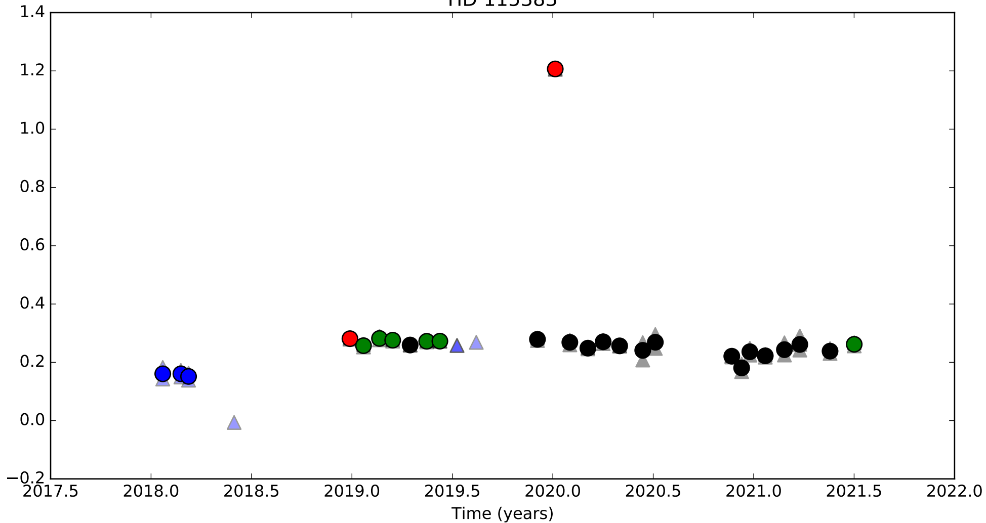
HD 115383
