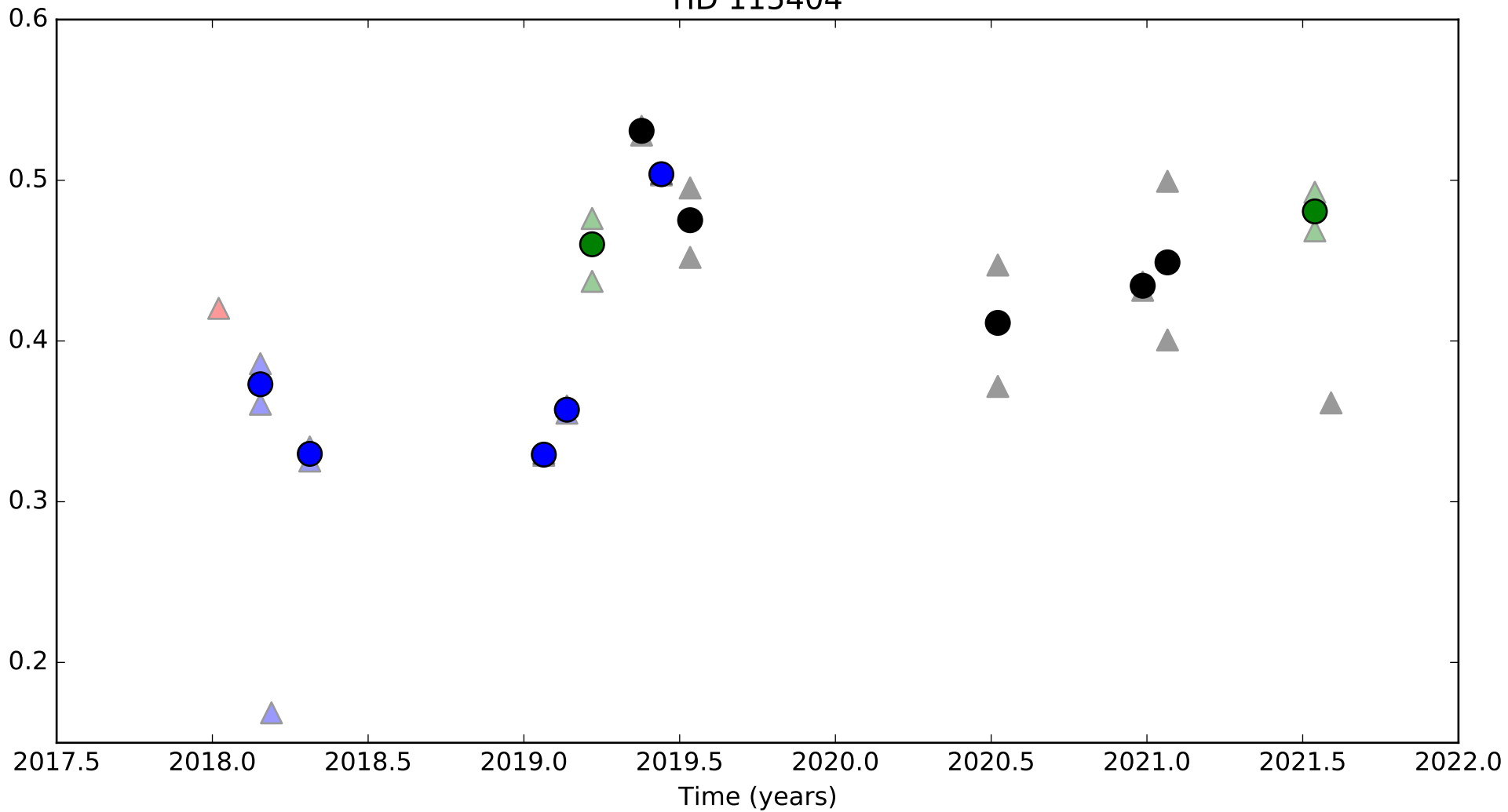
HD 115404
