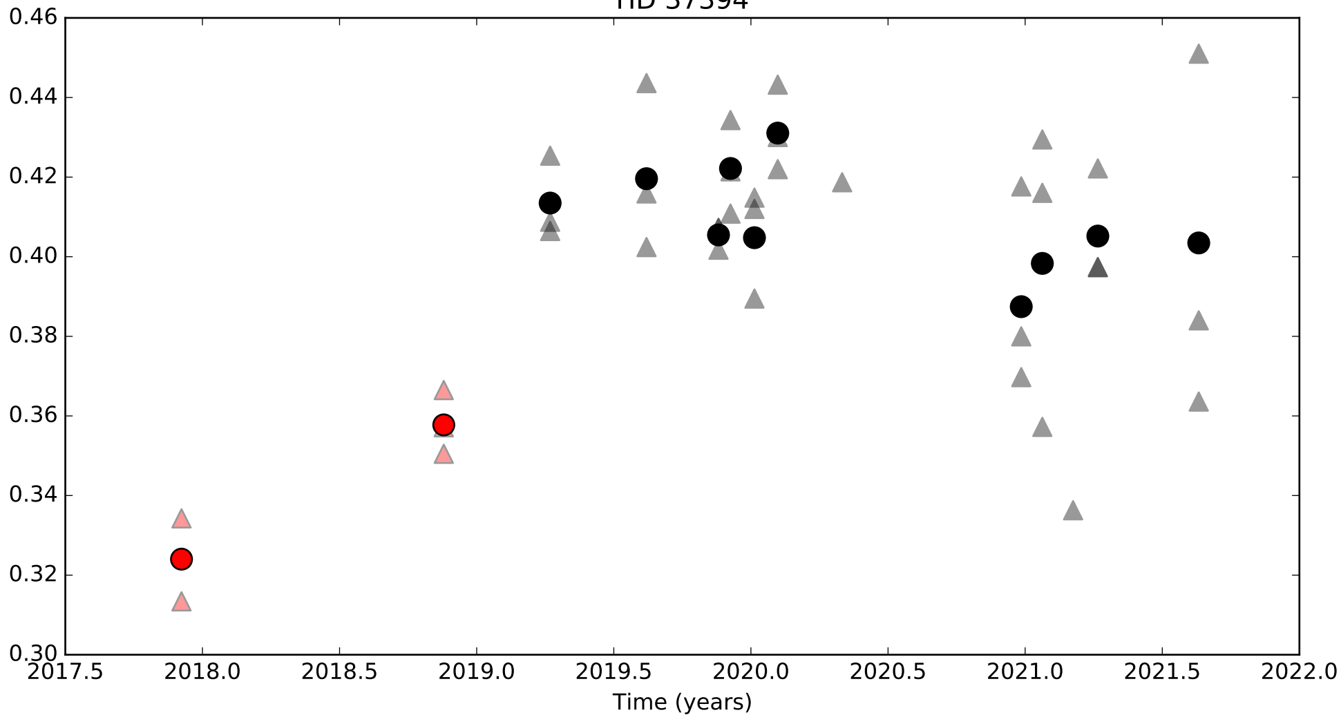
HD 37394
