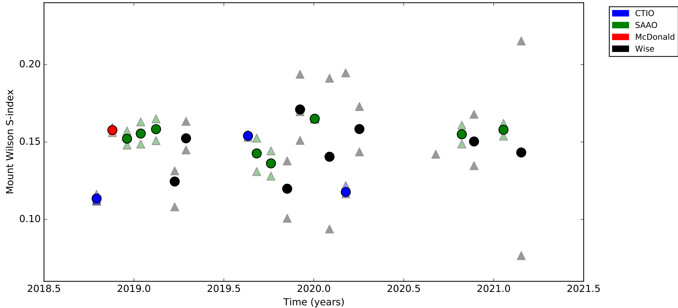
HD 49933
