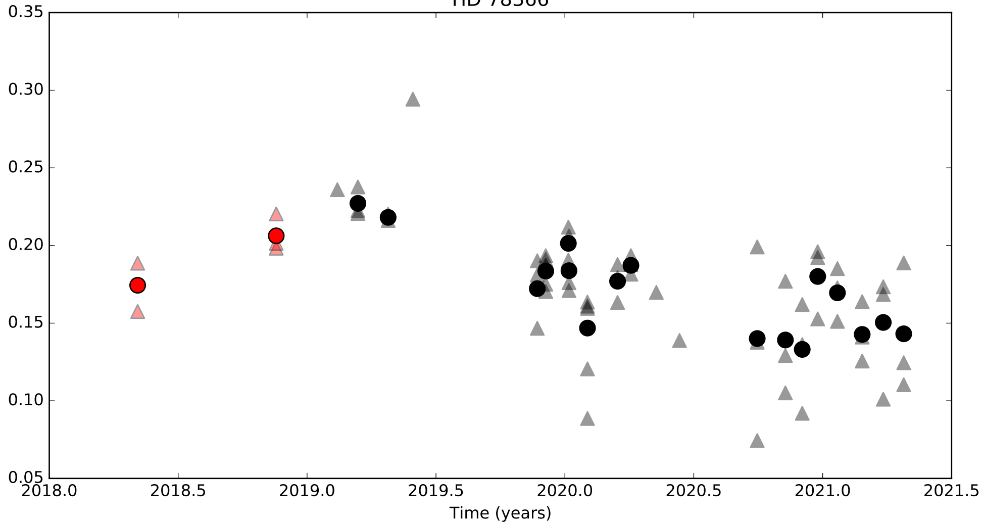
HD 78366
